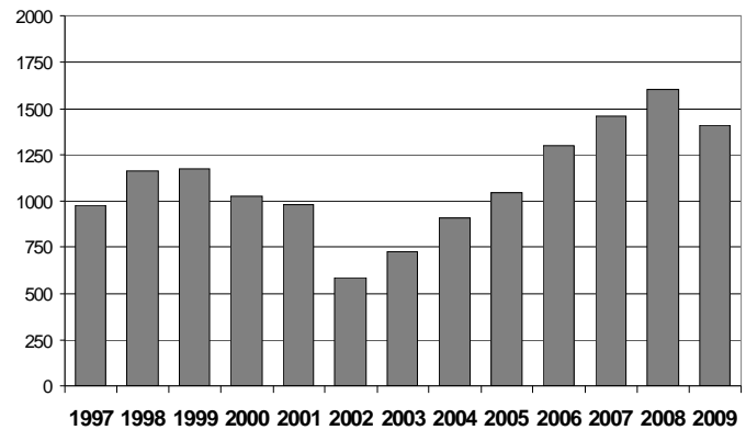
Gráfico 2. Despachos de cemento en miles de toneladas. Primer bimestre de cada año 1997/2009
